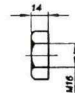
⑥ HEX NUT MATL. M.S. QTY. = 4 Nos.
